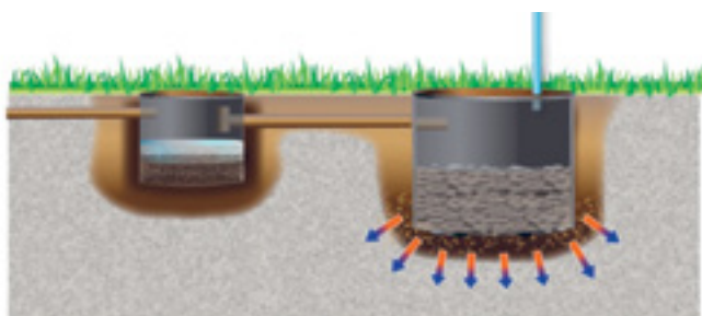
Imeytyskaivo pienille, rasvaisille pesuvesille, sako-osalla.
